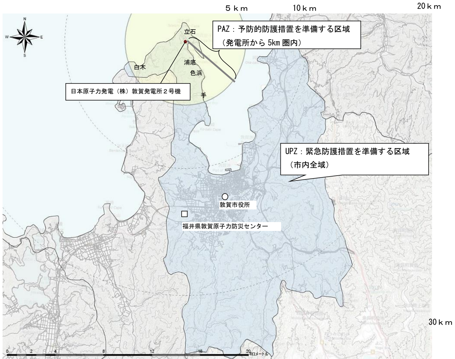
図 1 - 1 - 2 敦賀市において原子力災害対策を重点的に実施すべき地域の範囲
